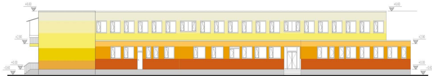
ФАСАДА СЕВЕР
